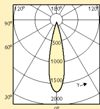
Křivky svítivosti
