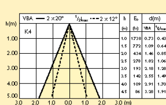
Vyzařovací diagram
