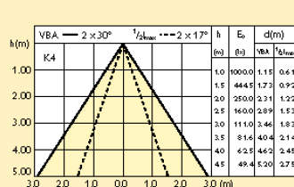
Vyzařovací diagram
