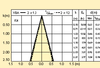
Vyzařovací diagram
