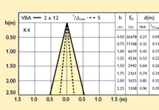
Vyzařovací diagram
