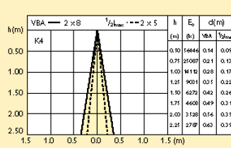
Vyzařovací diagram
