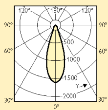
Křivky svítivosti
