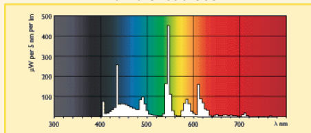
Barva světla 835
