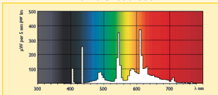
Barva světla 930
