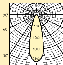
Křivky svítivosti
