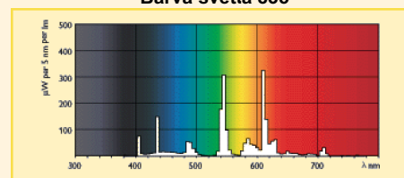
Barva světla 835
