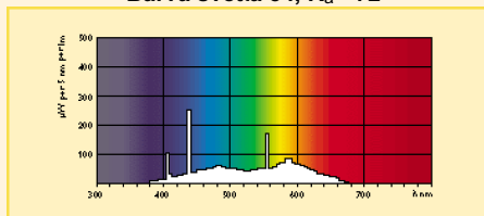
Barva světla 54, R_a = 72
