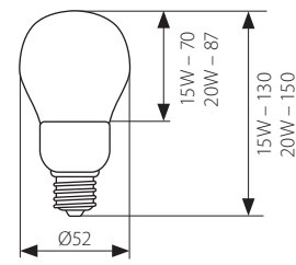
GLOB XEU48-...G
