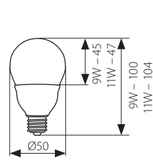
GLOB XEU48-...XG
