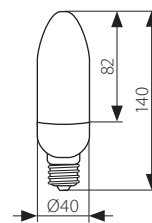
DART CDL-11S
