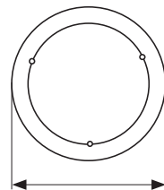
ARDEA 1030 MG/ML-SR – Ø260 ARDEA 1030 SG/ML-SR – Ø310 ARDEA 1130 DG/ML-SR – Ø375
