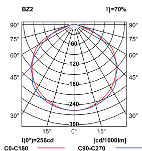
křivky svítivosti / krivky svietivosti
