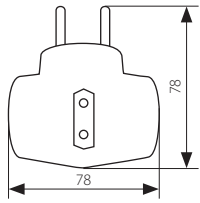
ZARK KRT/2-1
