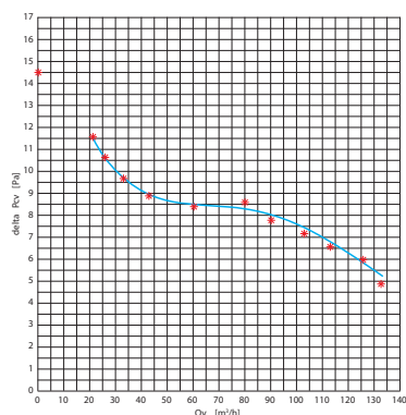
Charakteristika ventilátoru Charakteristika ventilátora
