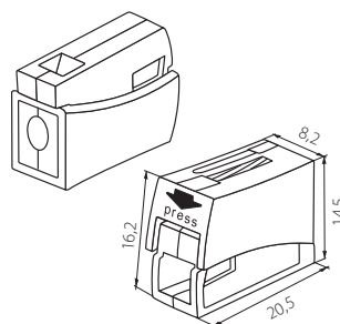
PC 301/PA
