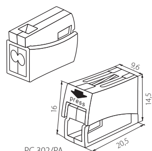
PC 302/PA
