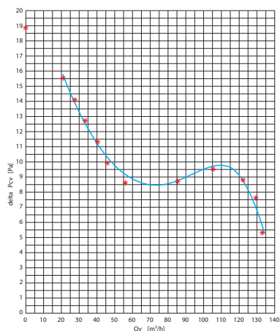
Charakteristika ventilátoru Charakteristika ventilátora
