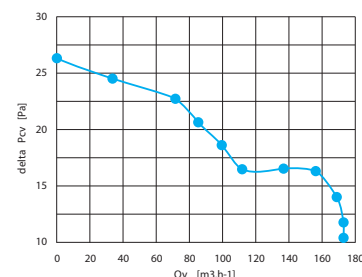
Charakteristika ventilátoru Charakteristika ventilátoru
