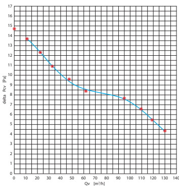
Charakteristika ventilátoru Charakteristika ventilátora
