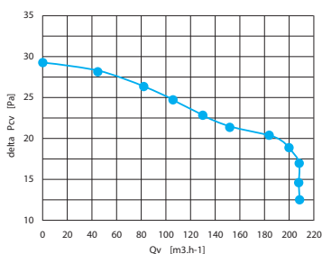
Charakteristika ventilátoru Charakteristika ventilátora
