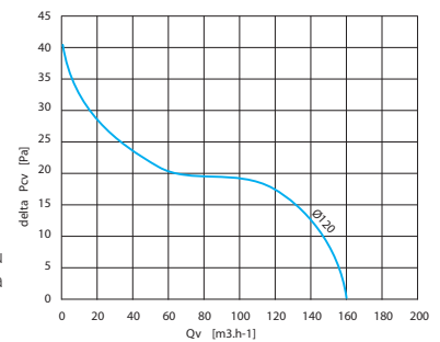
Charakteristika ventilátoru Charakteristika ventilátora
